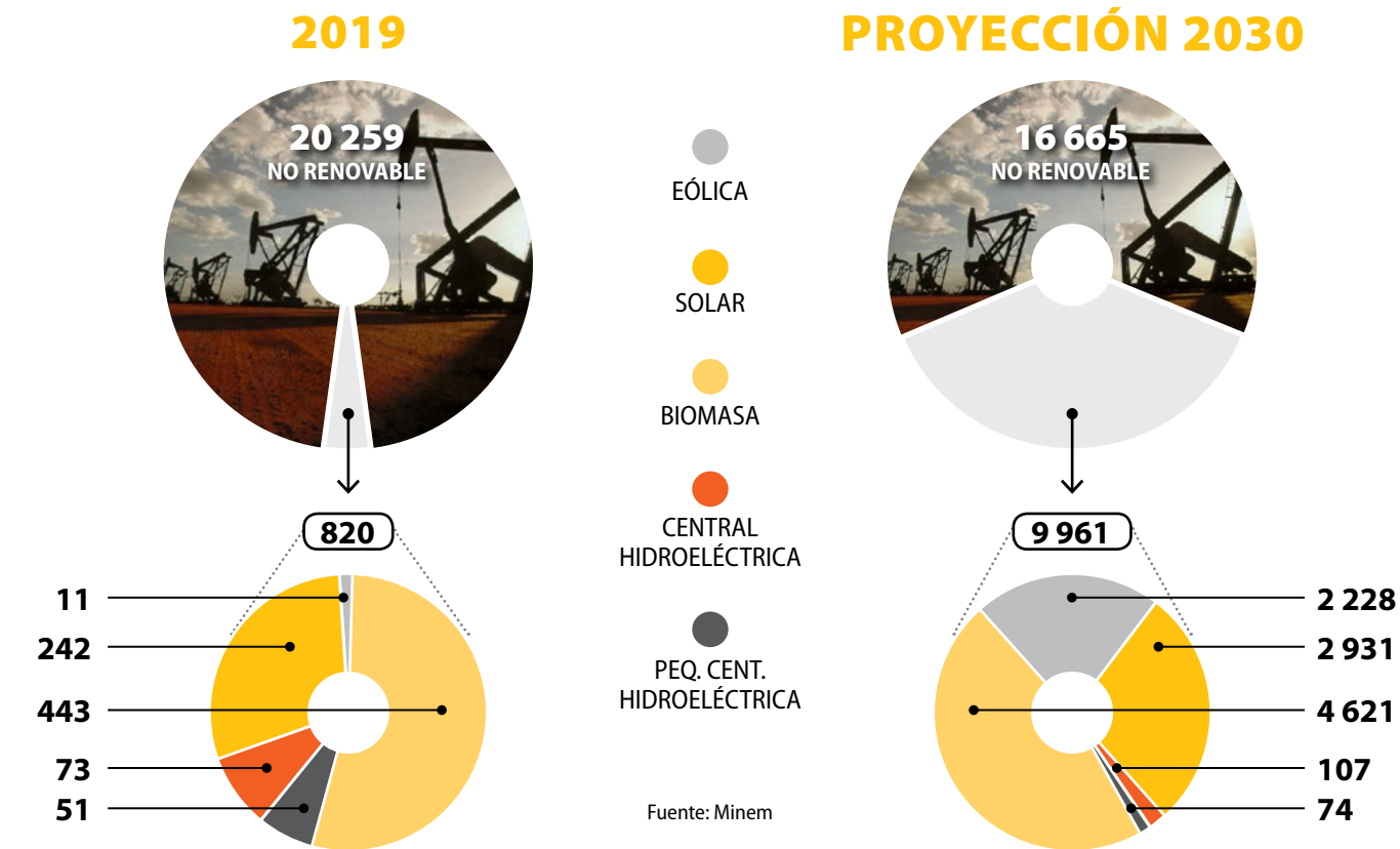
GRÁFICO III.7.3. GENERACIÓN CON FRE (GWh)
