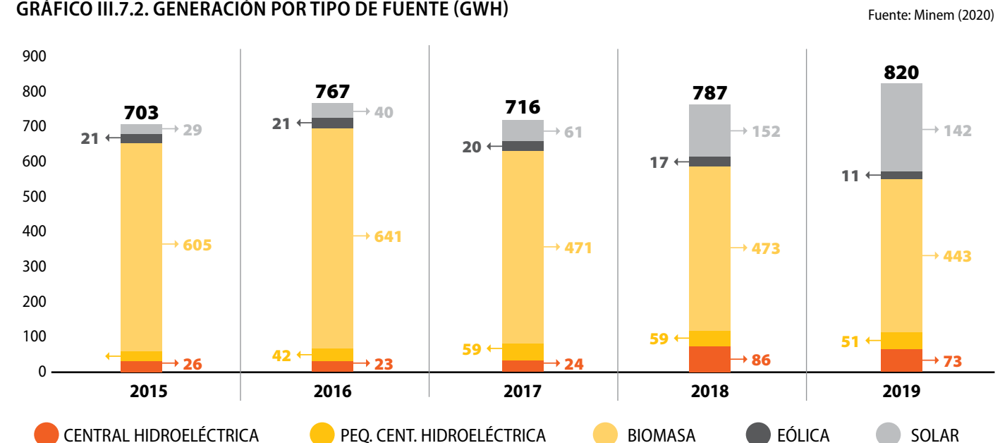
GRÁFICO III.7.2. GENERACIÓN POR TIPO DE FUENTE (GWH)
