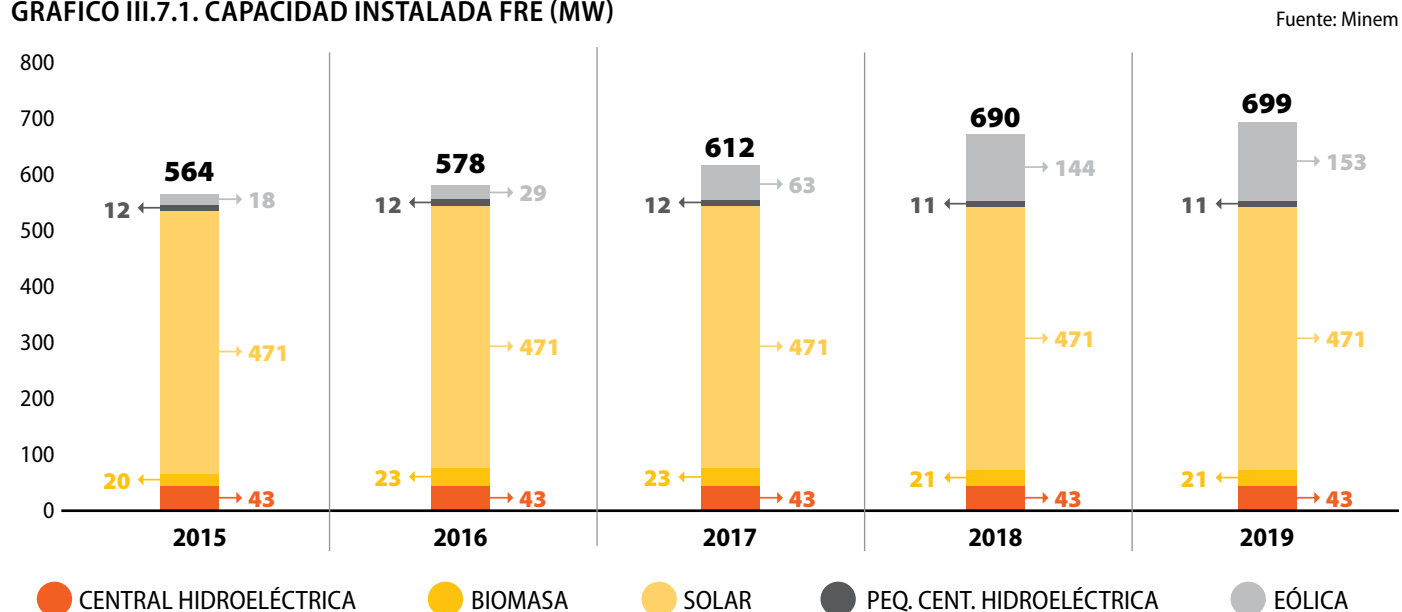
GRÁFICO III.7.1. CAPACIDAD INSTALADA FRE (MW)
